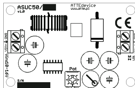
Rys.1. Widok płyty modułu ASUC50.
