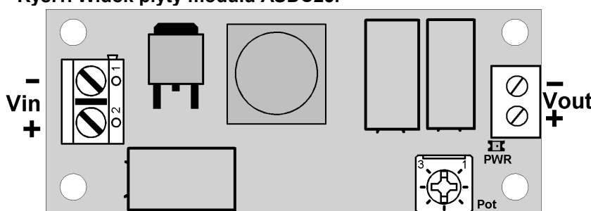
Rys.1. Widok płyty modułu ASDC25.
