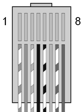
Rys.2. Prawidłowe zaciśnięcie przewodów we wtyku RJ-45 (standard T568B).
