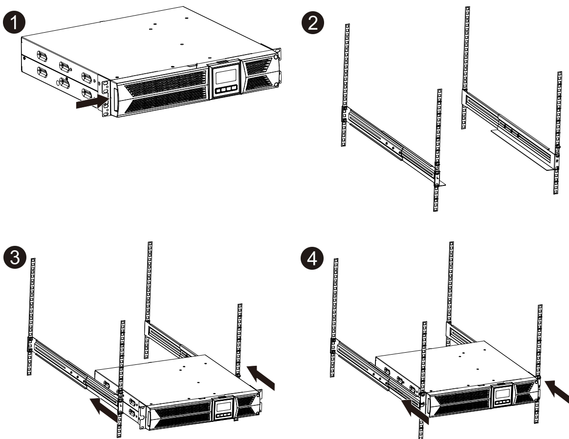
Rys. 2 Montaż Rack
