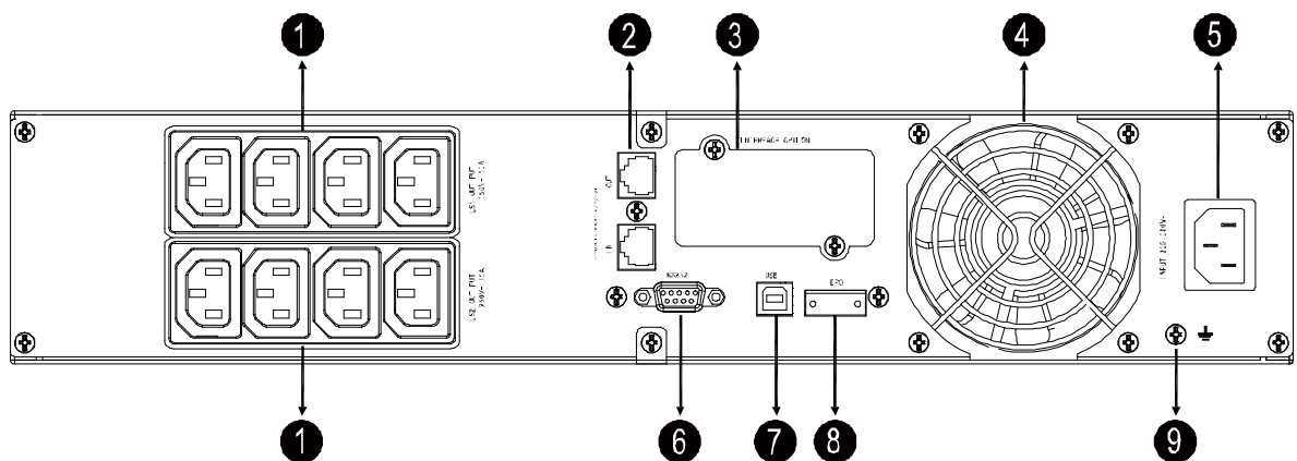
Rys. 8 Panel tylny UPS GT M 2K
